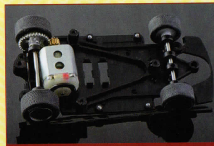
Detalle chasis
